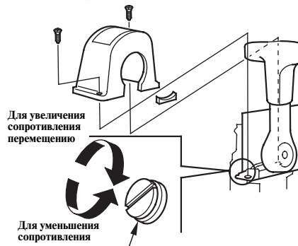
РЫЧАГ УПРАВЛЕНИЯ ФРИКЦИОННОГО ДЕМПФЕРА
