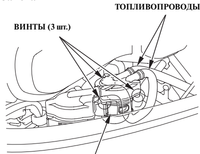
ЛЕНТОЧНЫЙ ХОМУТ
