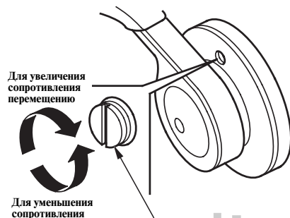
РЫЧАГ УПРАВЛЕНИЯ ФРИКЦИОННОГО ДЕМПФЕРА
